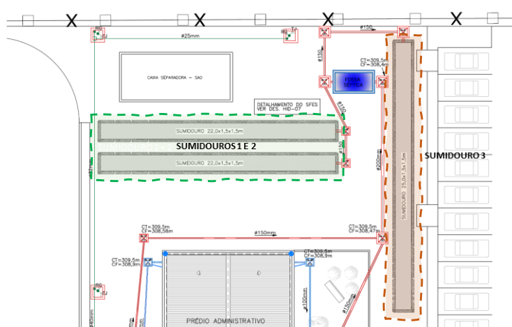
Figura 15. Projeto Sumidouro Exemplificativo. Fonte: elaboração própria.
