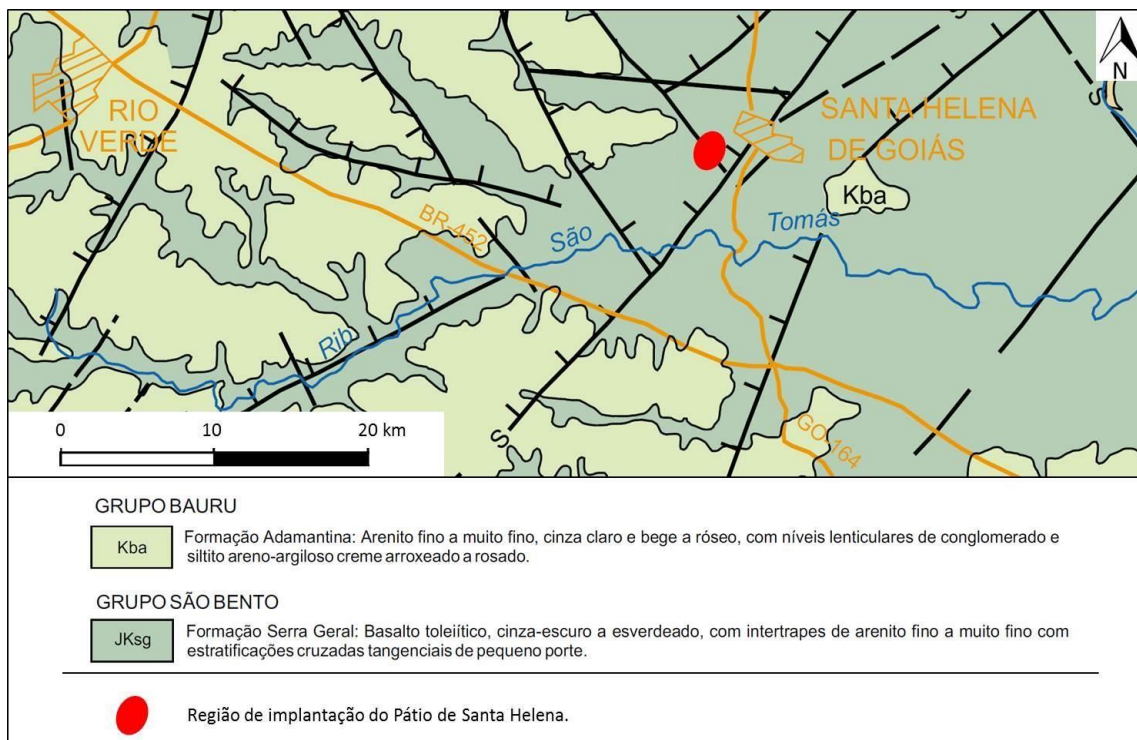
Figura 2. Mapa Geológico da região de implantação do novo traçado do Pátio.
